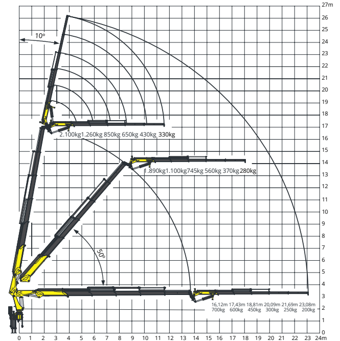
Gráfico de carga com Fly-jib
